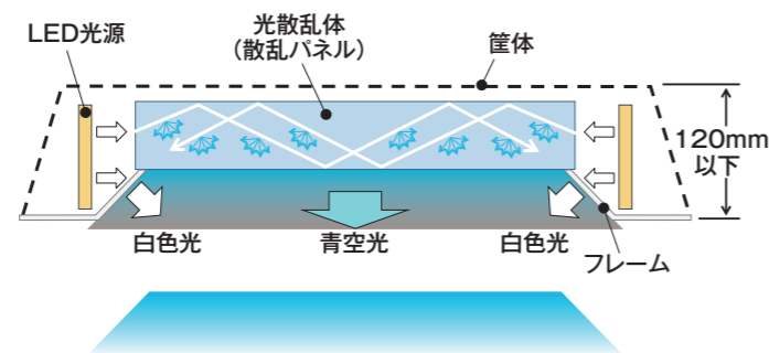
散乱パネルとフレームの組合せで奥行き感のある青色を演出しながら独自の薄型構造を実現した
